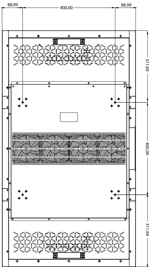
СХЕМА ДИСПЛЕЯ (ВИД СЗАДИ)
